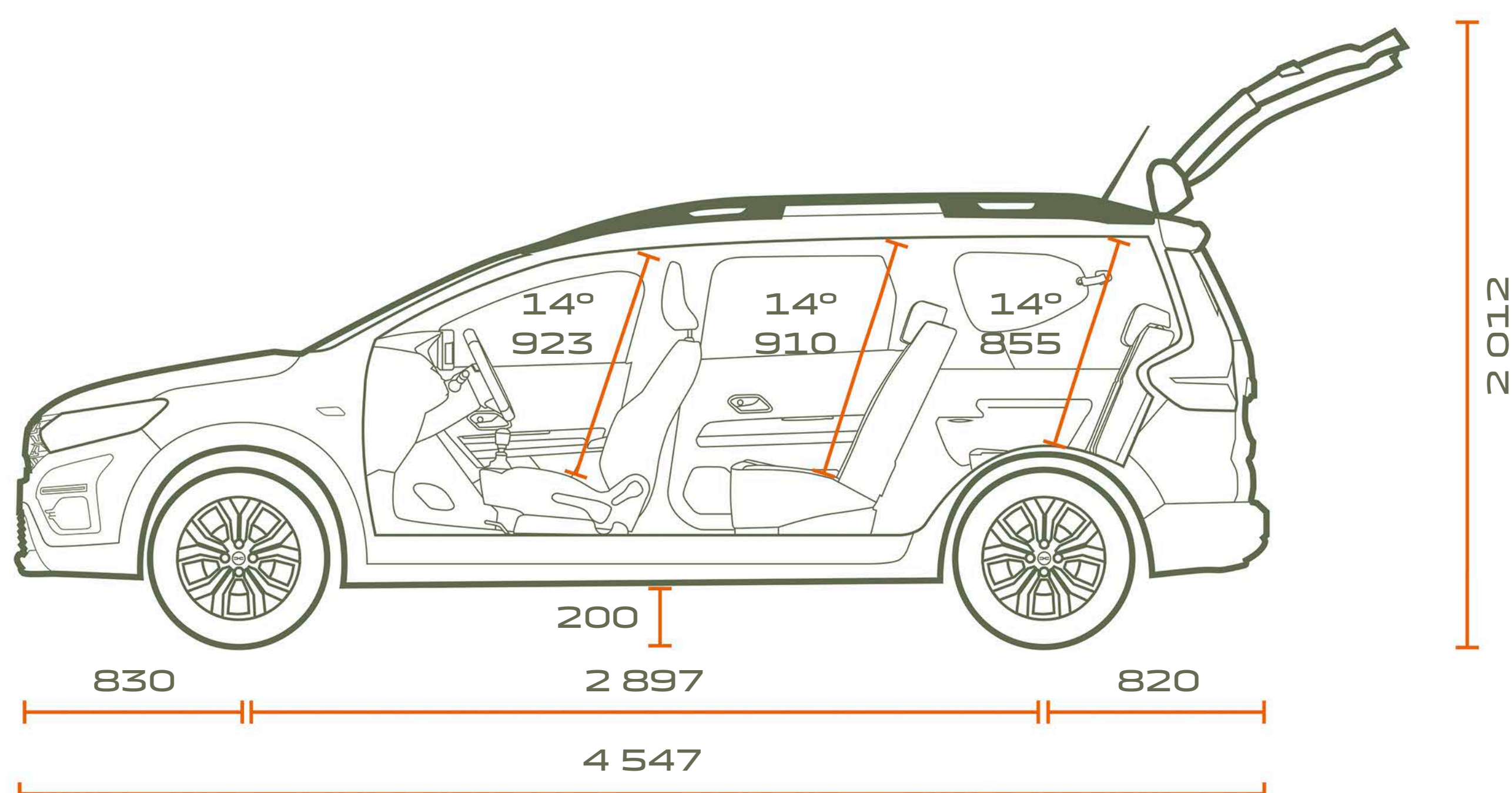
7 ÜLÉSES OLDALNÉZET
