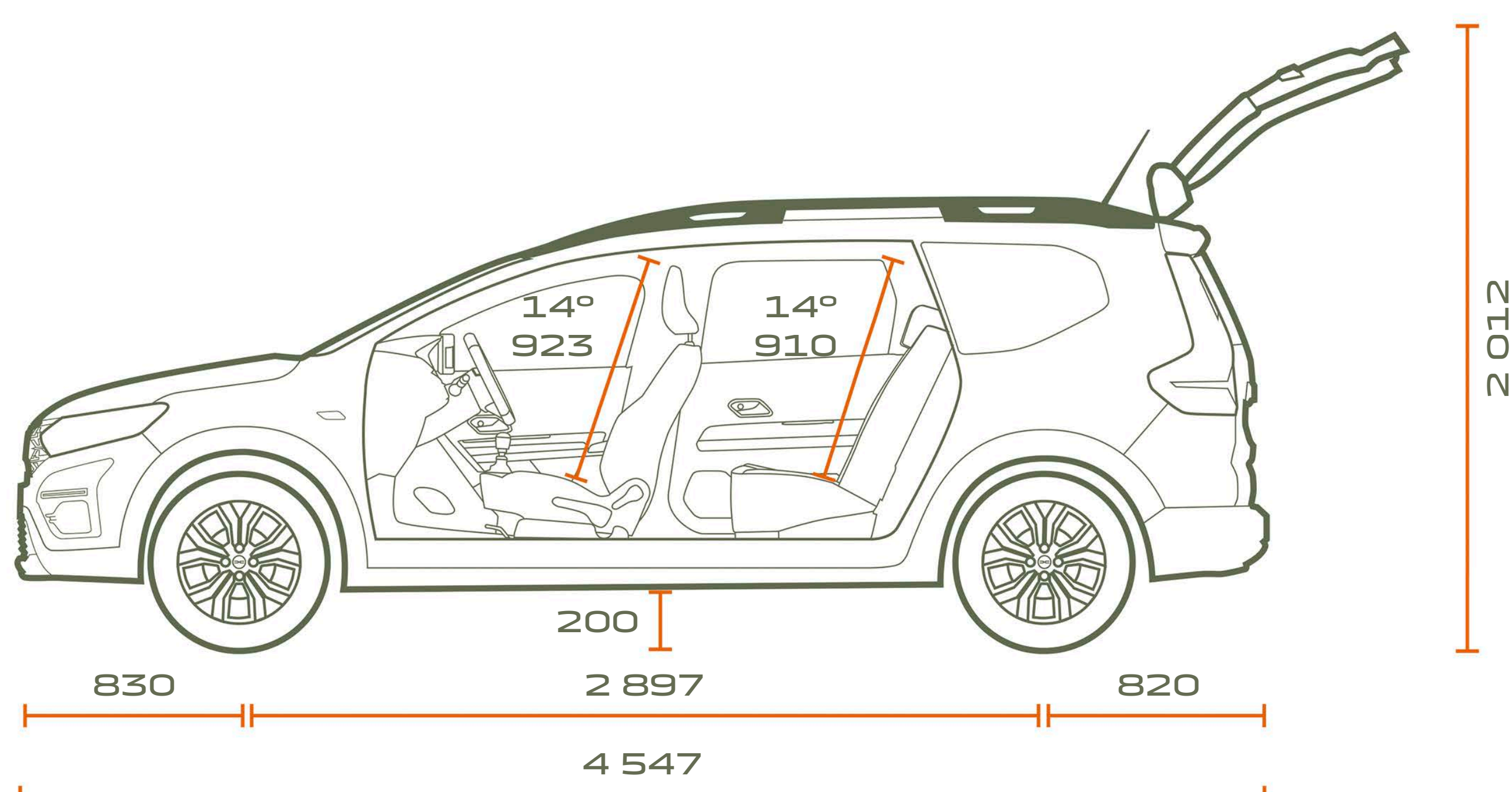
5 ÜLÉSES OLDALNÉZET
